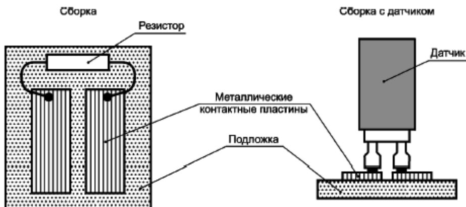
Рисунок 3 - Сборка для проверки сопротивления
